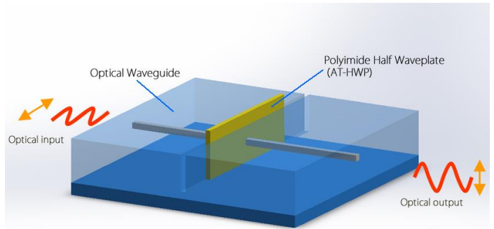
ポリイミド波長板を挿入した偏波モードコンバータ
