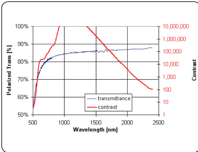
Fig. 1-10 Ultra-High Contrast IR Polarizer
